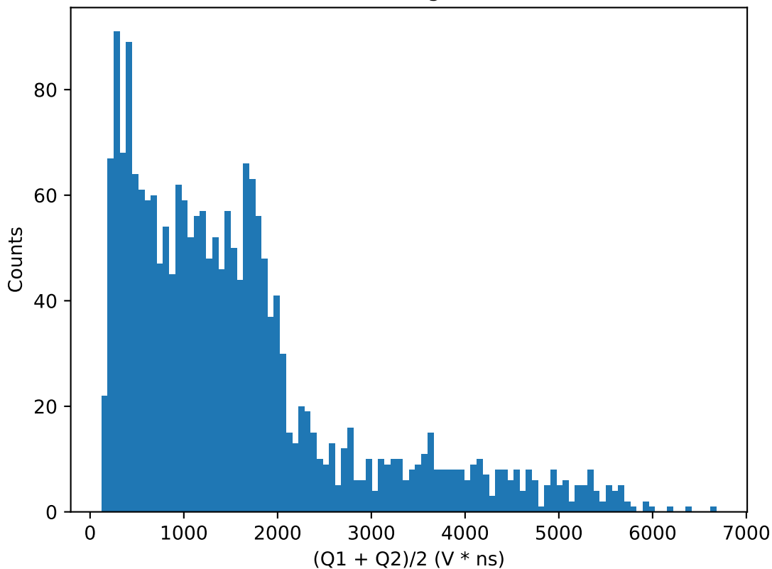
(Q1 + Q2)/2 histogram for 44.5V
